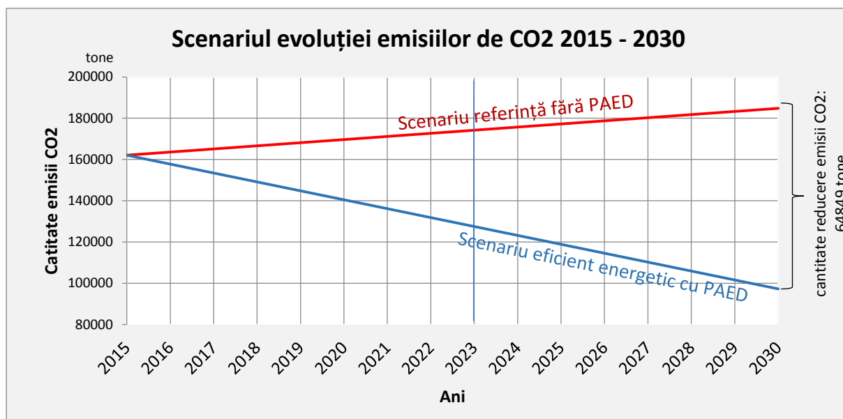
Figura 70. Scenariul evoluției emisiilor de CO 2 , 2015-2030.
